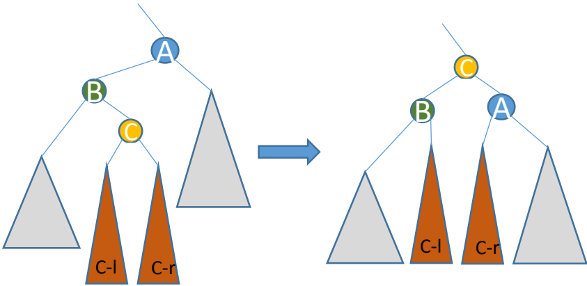
Left-Right Rotation
