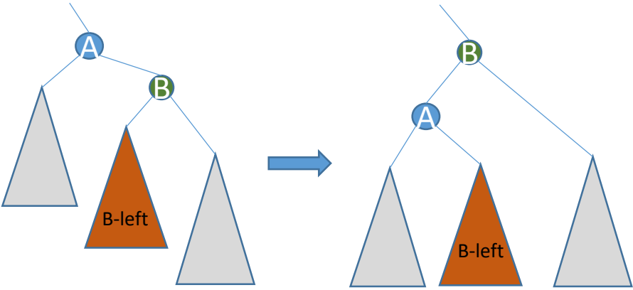
Left Rotation
